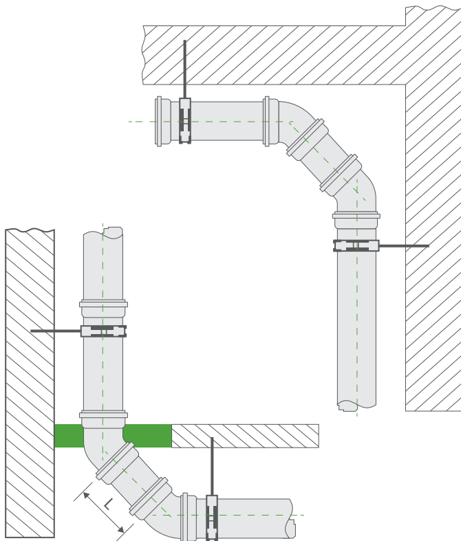
شکل ۱۱ ثبات سیستم فاضلابی در محل‌های چرخش
