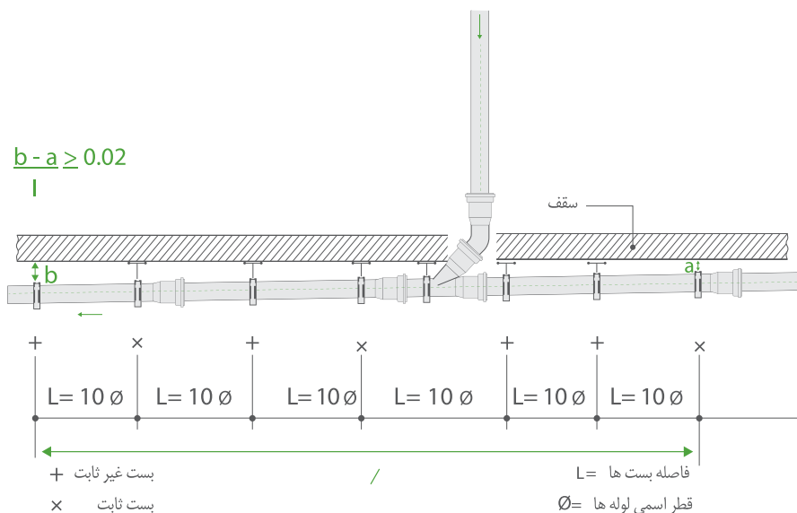
روند استفاده از بسته‌های ثابت و غیر ثابت در سیستم فاضلاب
